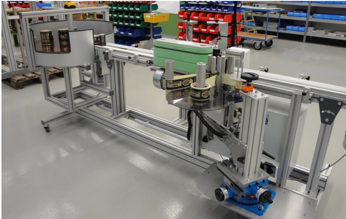
Transportband mit Etikettenspender EcoLine 100-XS im Liegenbetrieb, Rundum Etikettier Station und Auslaufdrehteller.
